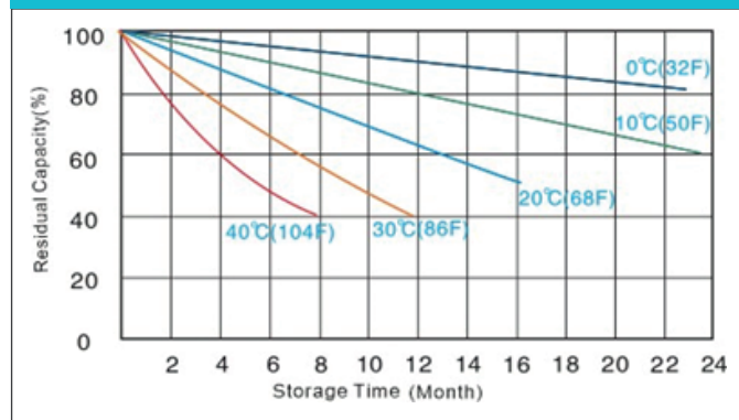
Характеристики хранения
